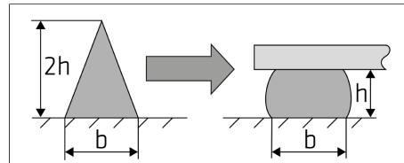
Kuva 1: Ohje liimasauman levitysmuodoksi ja puristamiseksi lopulliseen muotoon.
